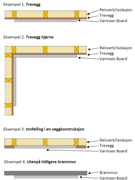
Fig.1 Montering av Varmsen Board som brannmur.
