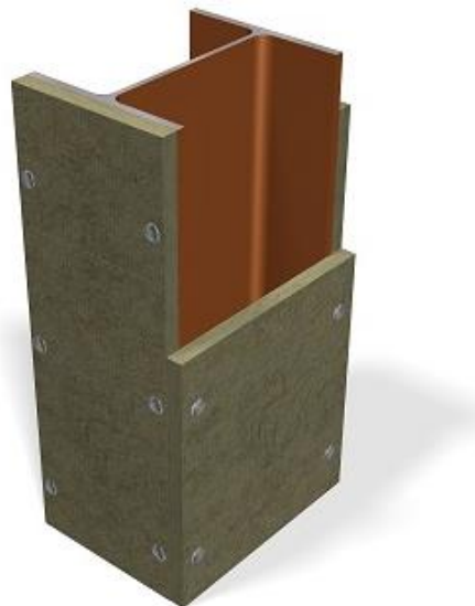
Fig.1 Protecta A-Plate.
